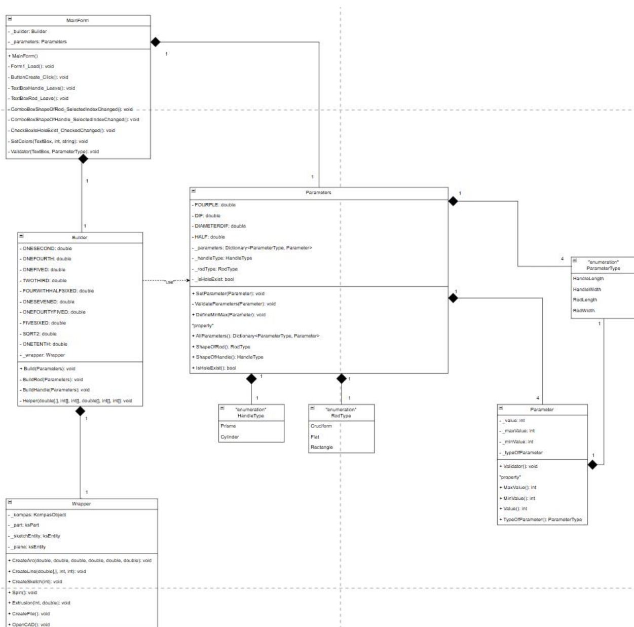
Рисунок 7.2 – UML диаграмма классов после реализации плагина «Отвёртка»
